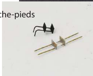
Voir les perçages sur les jupes pour le positionnement des marche-pieds
