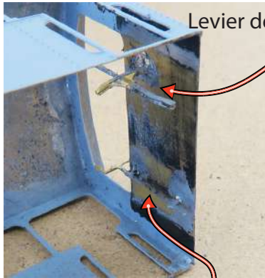
Manivelle de frein à gauche
